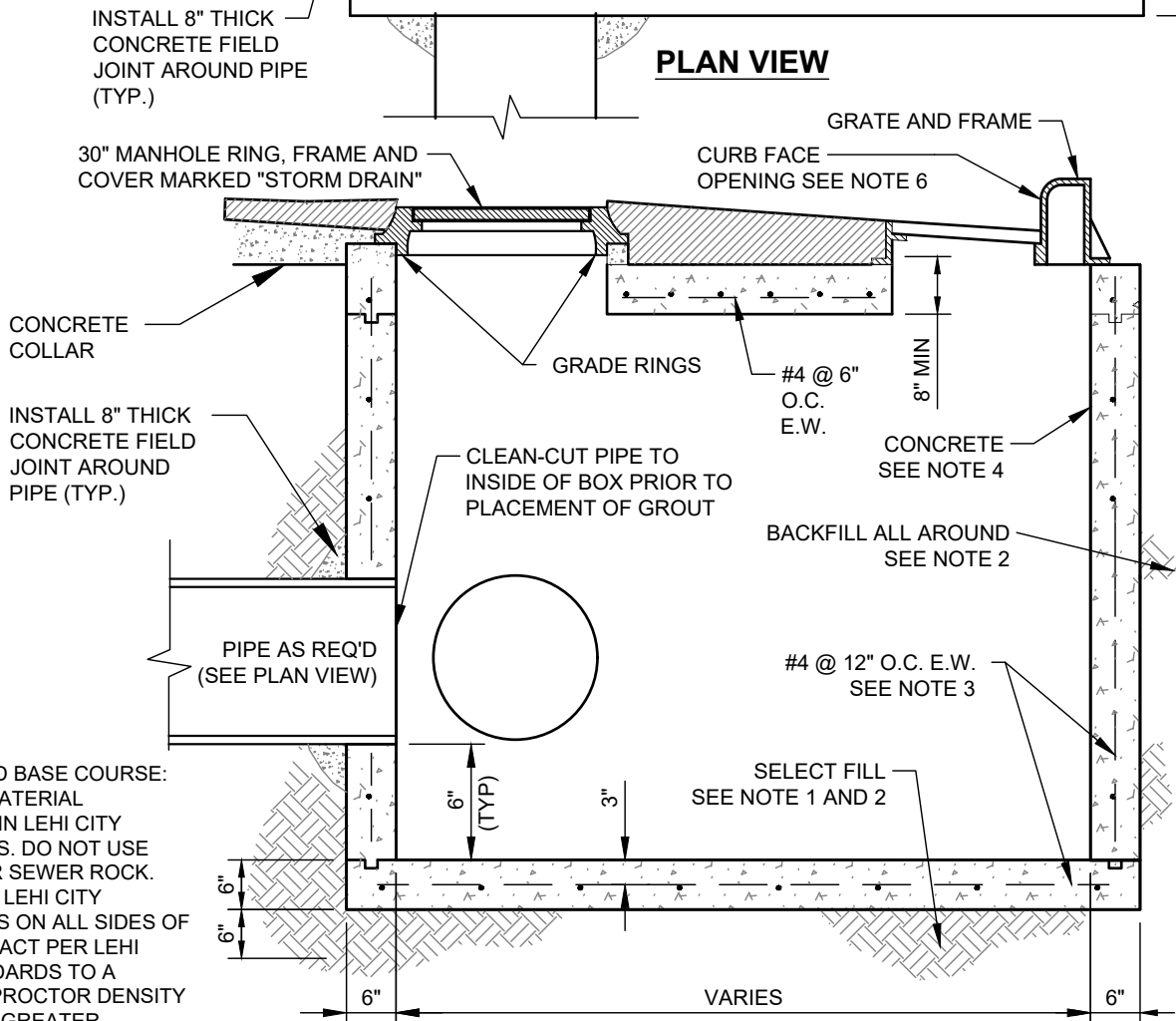
SECTION A-A
